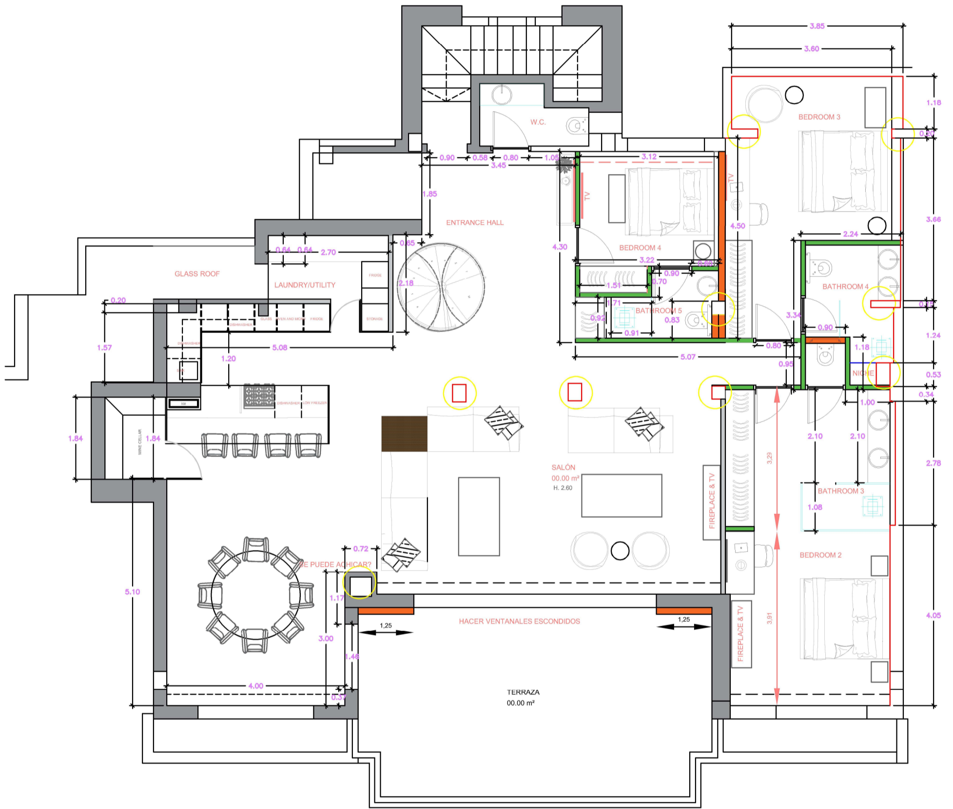
LAYOUT 4 - 25.02.23 PLANTA BAJA
