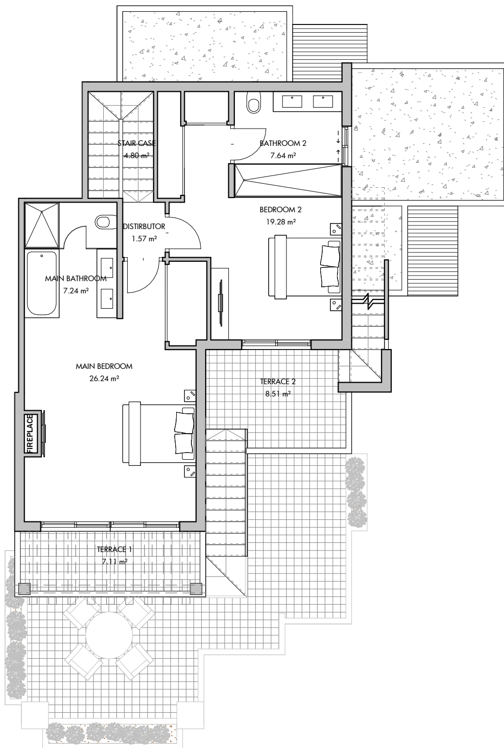
FLOOR 1°
